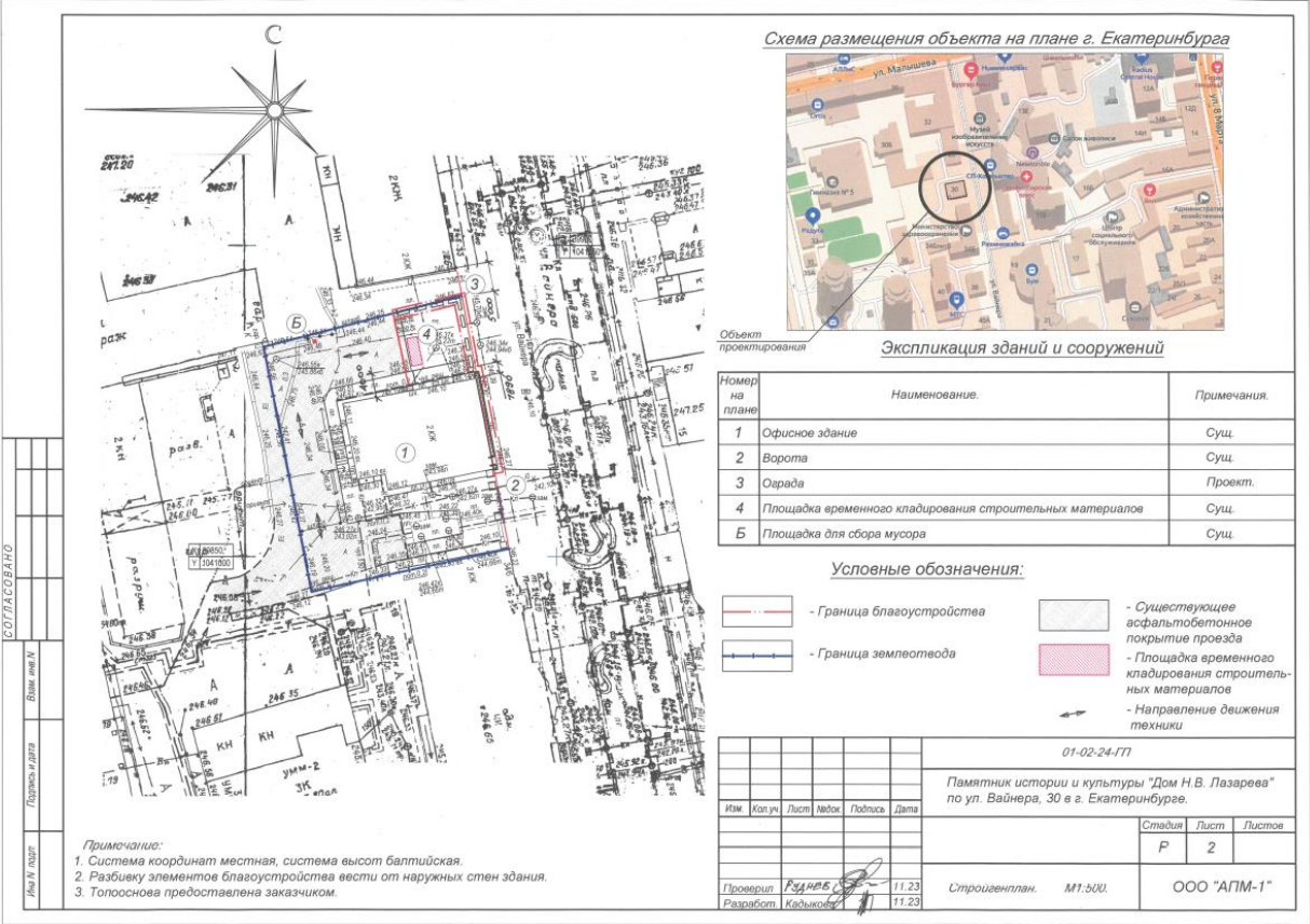
Стройгенплан. Забор объекта культурного наследия «Дом Н.В.Лазарева» по ул. Вайнера, 30 в г. Екатеринбурге
