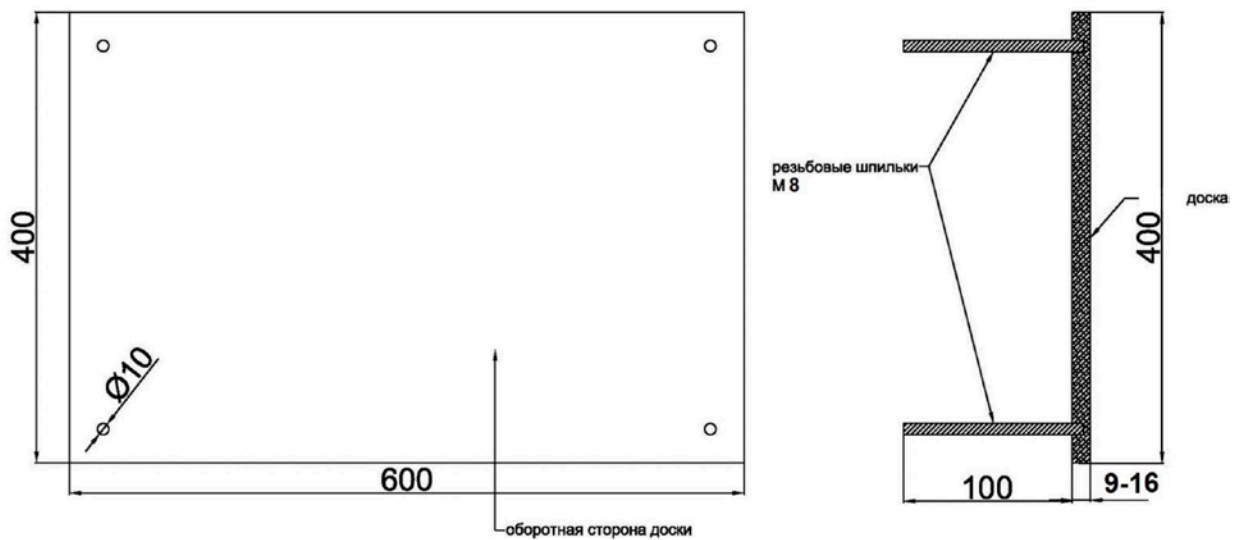
Рисунок 2. Схема крепления доски (пластины)
