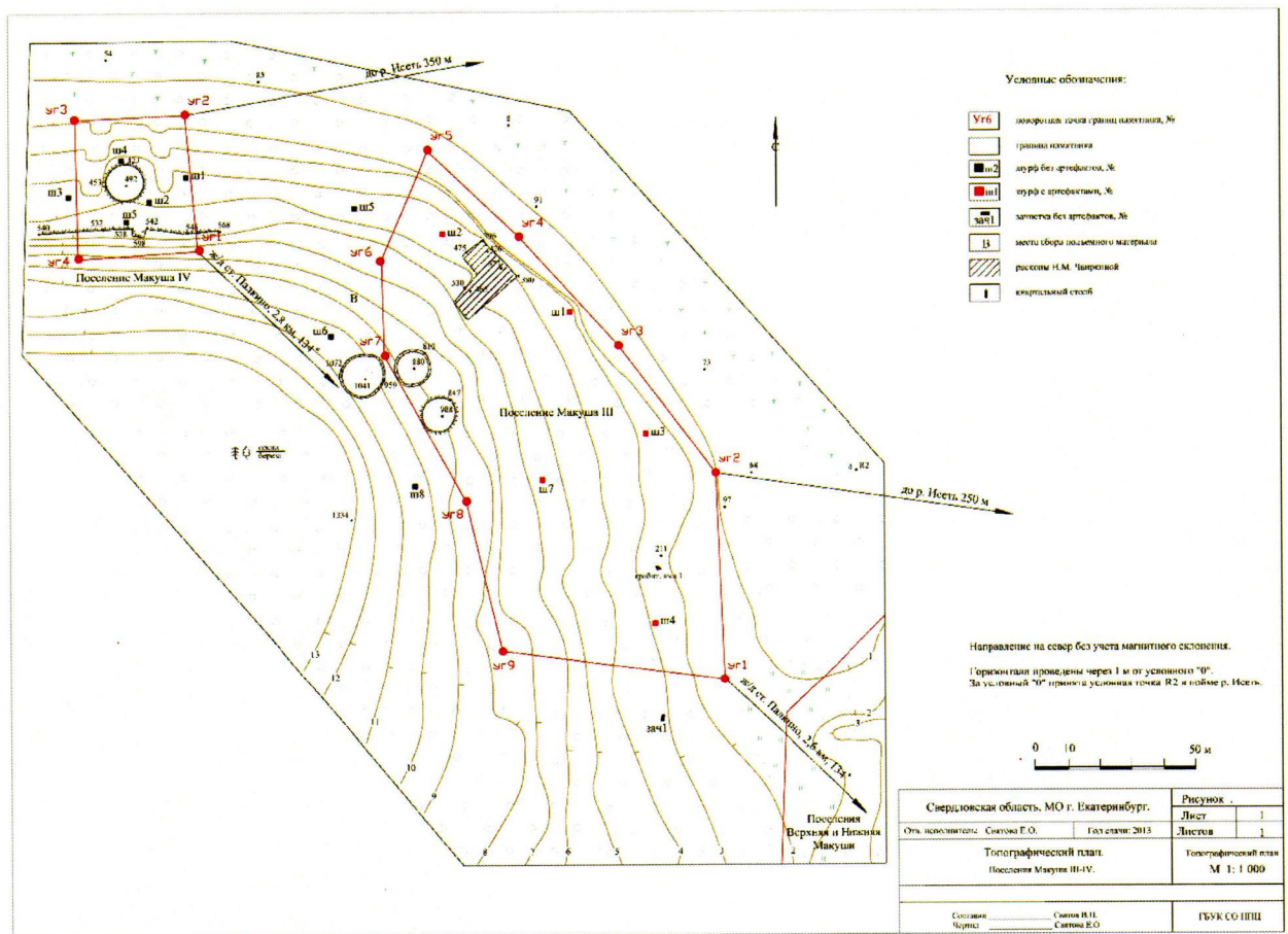
Топографический план объекта культурного наследия
