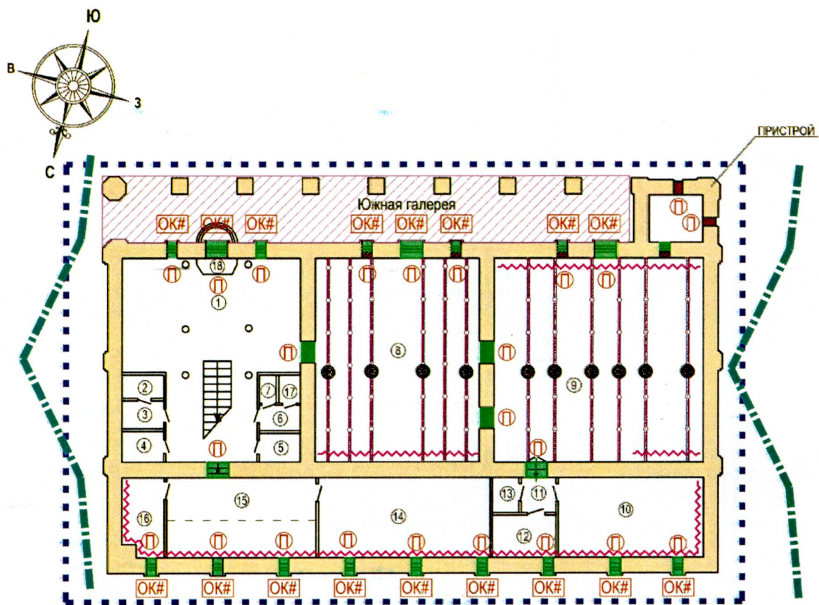
Схема предмета охраны объекта культурного наследия на плане первого этажа в уровне дверных проемов
