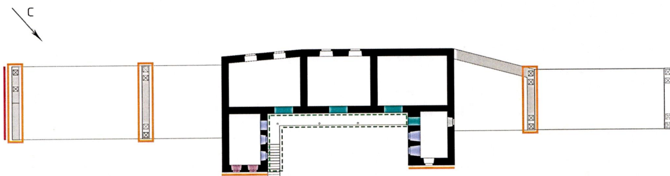
План второго этажа
