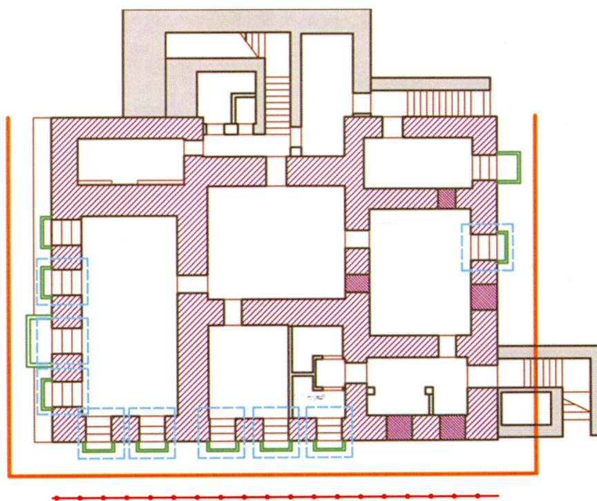
План цокольного этажа
