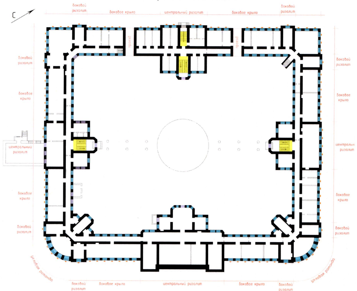
План цокольного этажа
