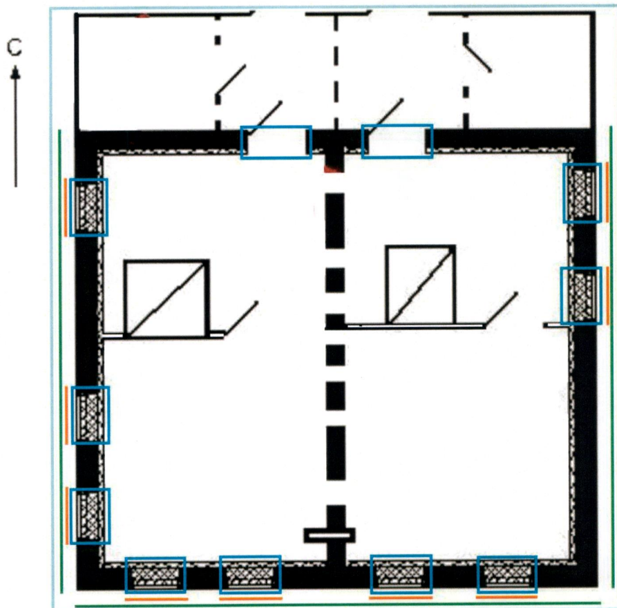
План цокольного этажа
