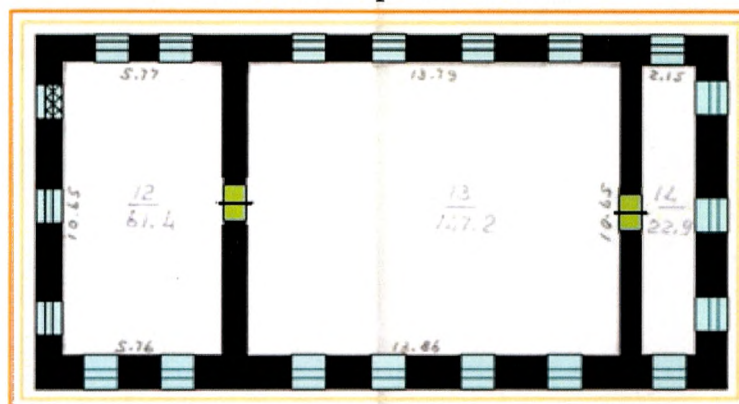
План пятого этажа
