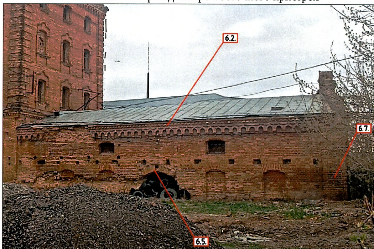
Юго-восточный фасад северо-восточного пристроя
